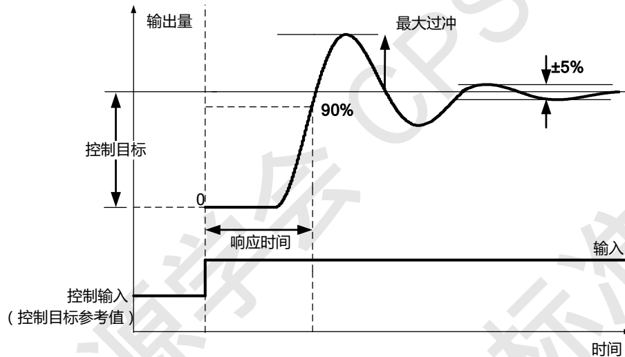
图1 响应时间示意图
